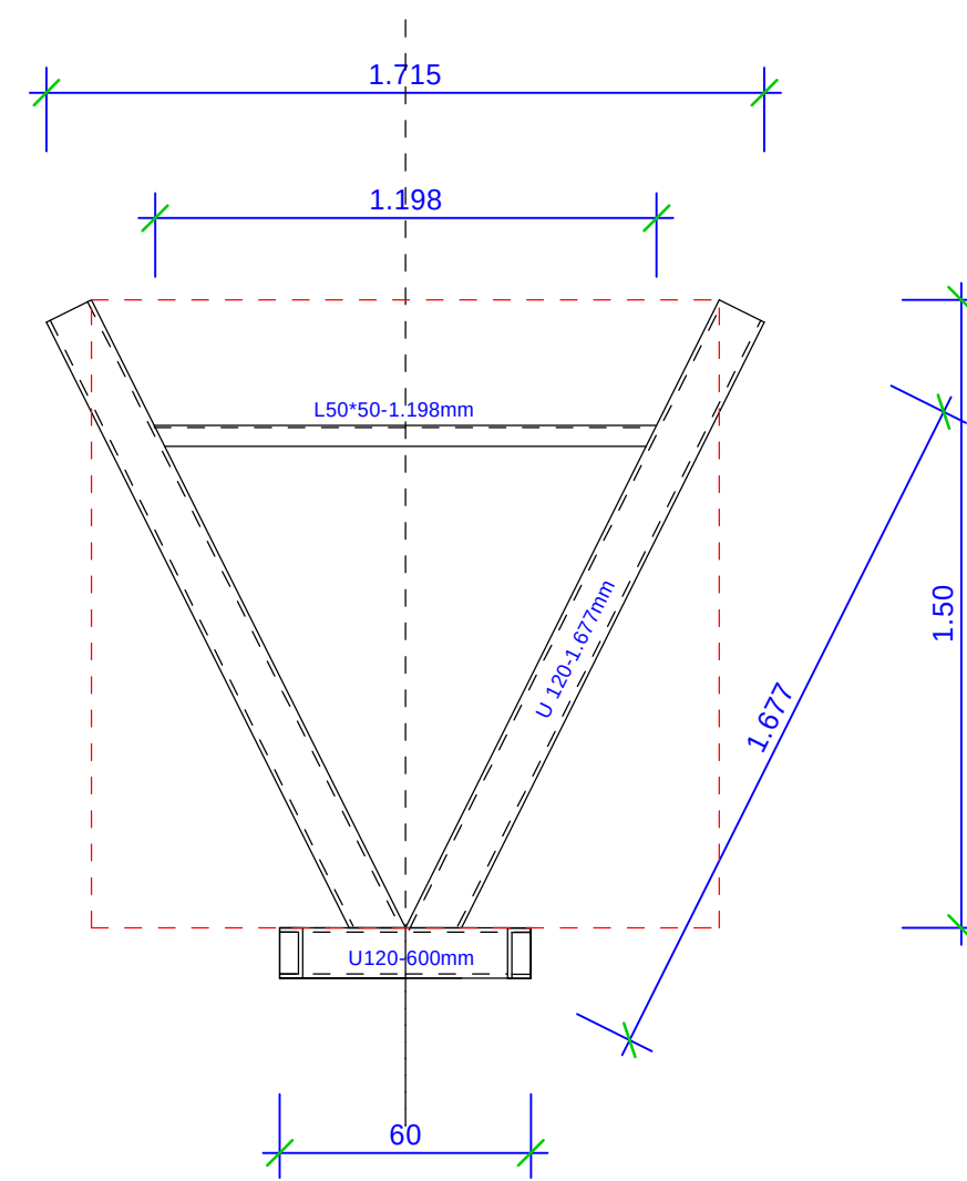
Draufsicht Untergestell
